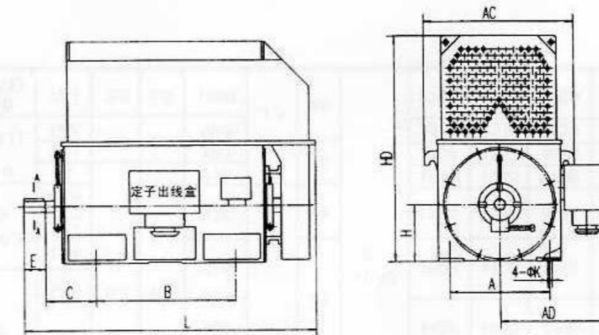
YKK355-500外形安装尺寸
