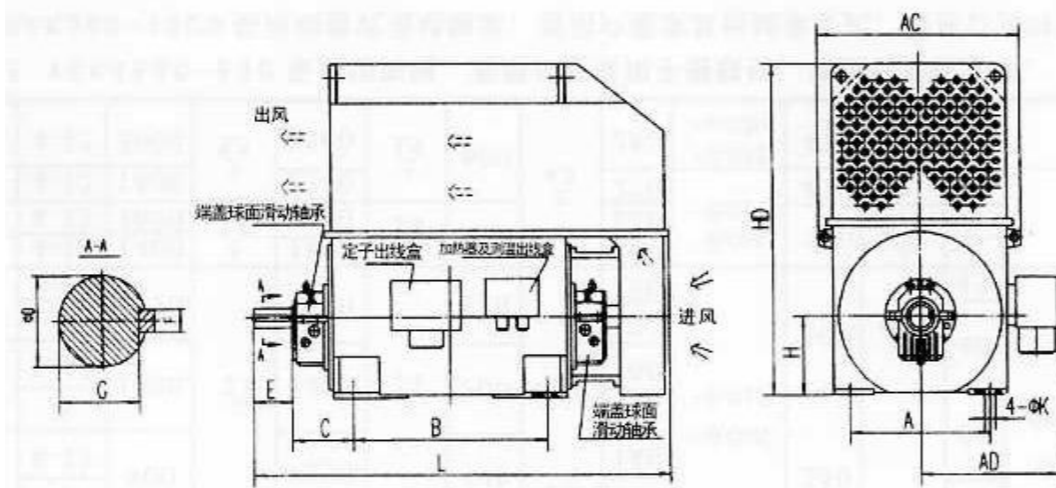
YKK560-1000外形安装尺寸
