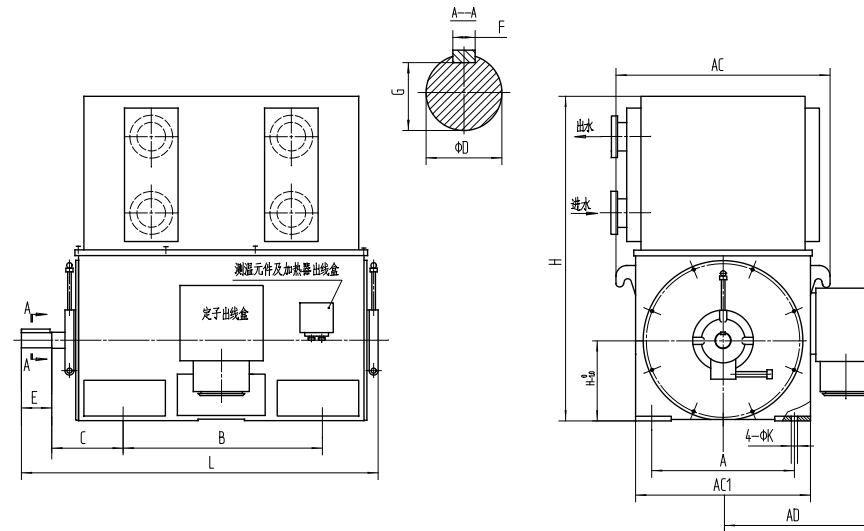
YKS355-500 安装尺寸表(6000V) YKS355-500 MOUNTING DIMENSIONS TABLE(6000V)
