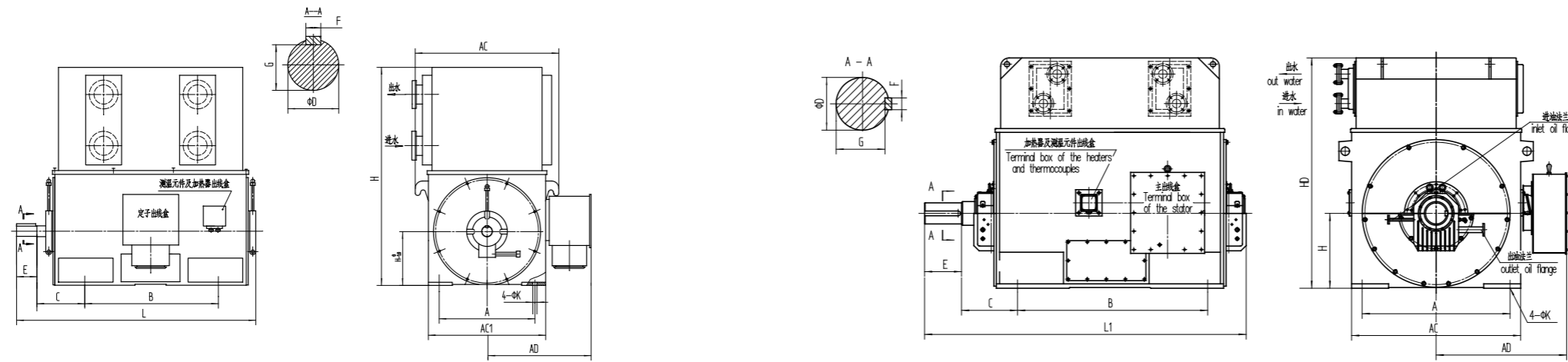
YKS450-1000 安装尺寸表(10000V) YKS450-1000 MOUNTING DIMENSIONS TABLE (10000V)
