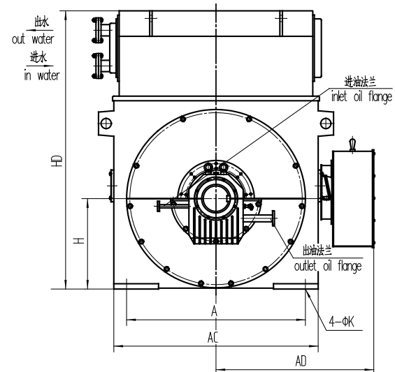
YKS560-1000 安装尺寸表(6000V) YKS560-1000 MOUNTING DIMENSIONS TABLE(6000V)
