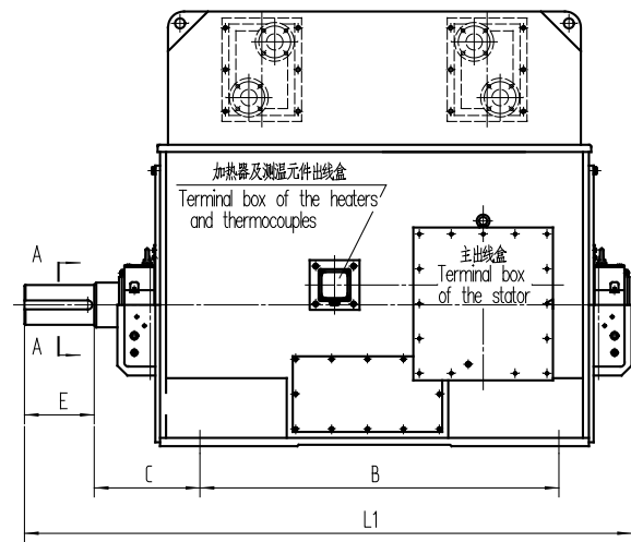
YKS560-1000 安装尺寸表(6000V) YKS560-1000 MOUNTING DIMENSIONS TABLE(6000V)
