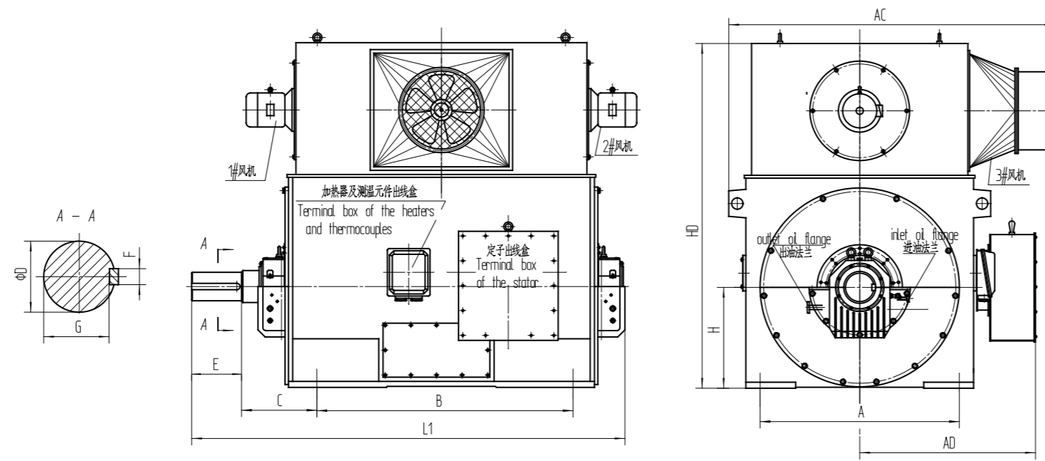
YPT560-1000 安装尺寸表(10000V) Y560-1000 MOUNTING DIMENSIONS TABLE (10000V)
