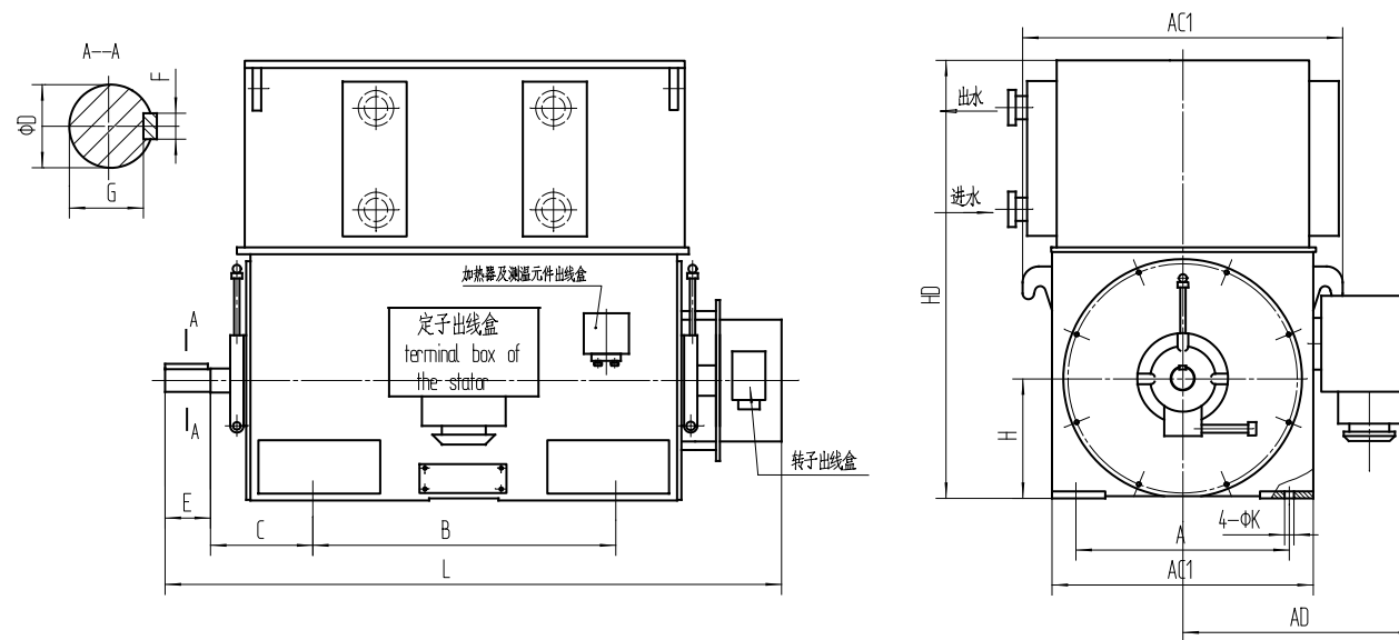
YRKS355-500 安装尺寸表(6000V) YRKS355-500 MOUNTING DIMENSIONS TABLE(6000V)
