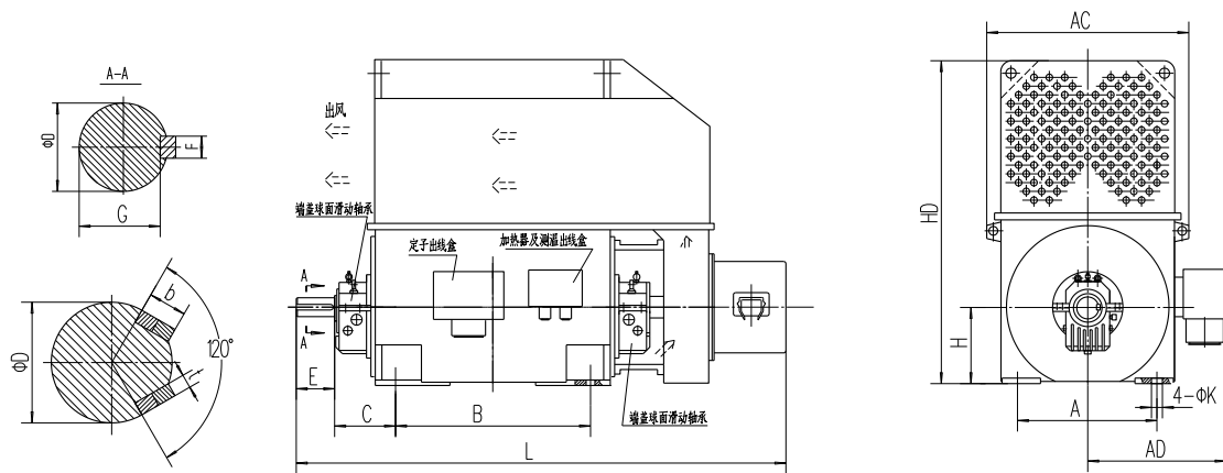
YRKK560-900外形安装尺寸
