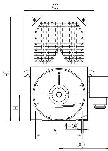
YKK450-500外形安装尺寸
