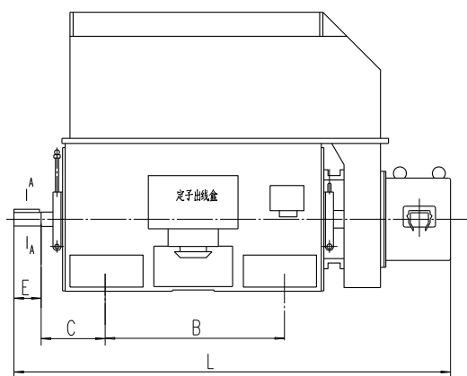
YRKK450-500外形安装尺寸
