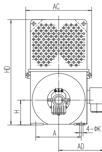
YKK450-500外形安装尺寸
