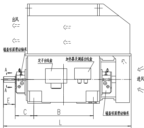
YKK450-500外形安装尺寸
