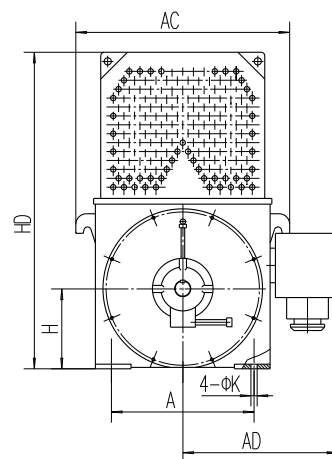
YKK560-900外形安装尺寸
